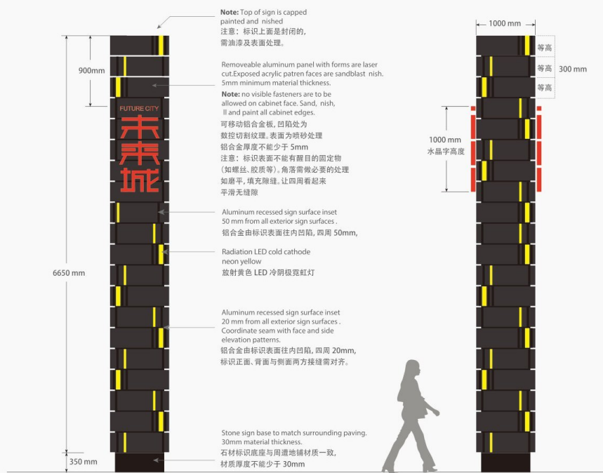
▲ 正视图 (Front view)
