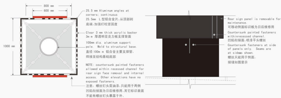
▲ 顶视图 (Top view)
