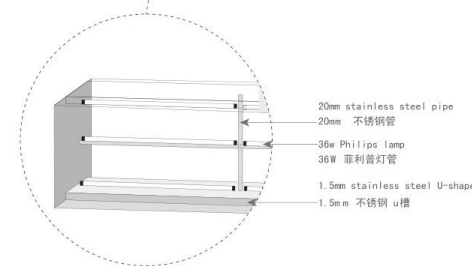
▲ 细节图 (Detail view)
