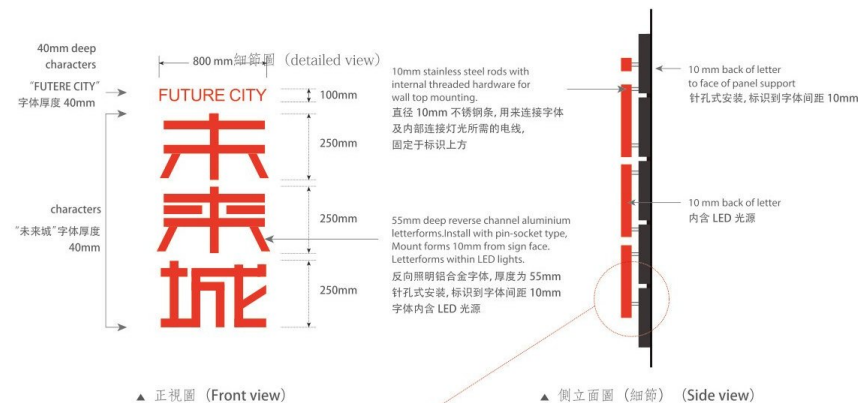
▲ 正视图 (Front view)
