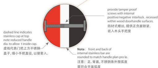
▲ 正视图 (Front view)
