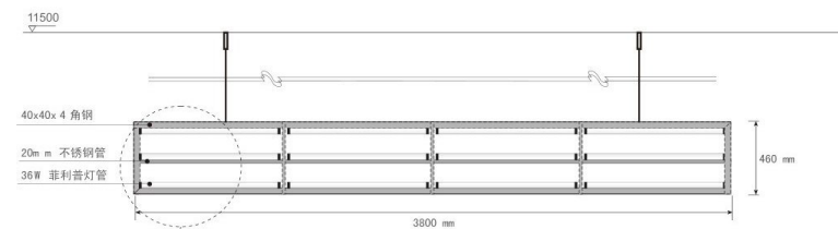
▲ 正视图 (Front view)
